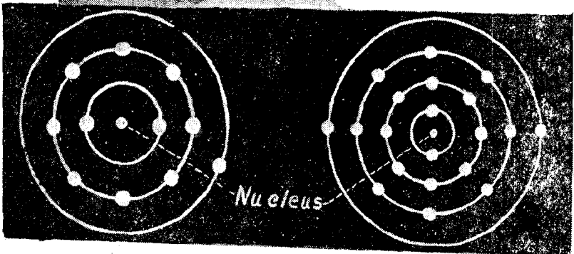
ఎడమవైపున ఉన్నది సోడియమ్ ఏటమ్. కుడివైపుది కార్బియమ్.
